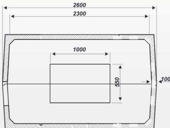
Przekrój poziomy
