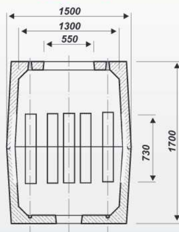
Przekrój poprzeczny
